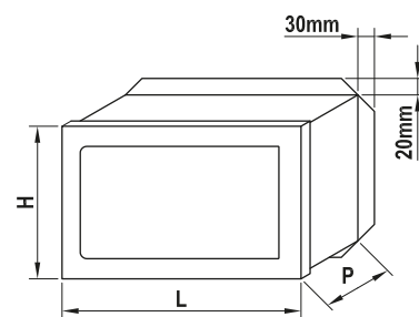
DETTAGLIO INGOMBRO ALETTE POSTERIORI ANTISTRAPPO CASSEFORTI A MURO
